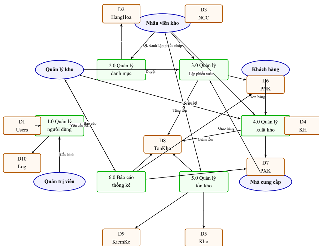
Hình 3.3: DFD cấp 1 – Phân rã các luồng dữ liệu trong hệ thống quản lý kho hàng
