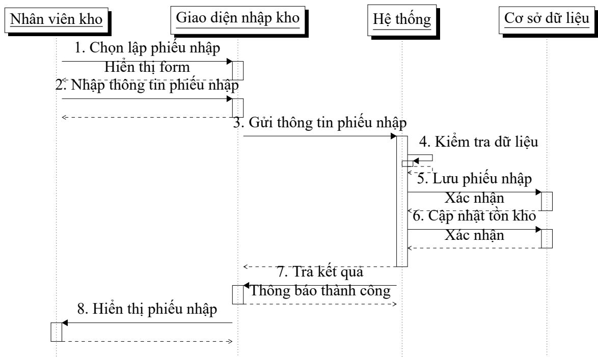
Hình 5.3: Sequence diagram UC09 – Lập phiếu nhập kho
