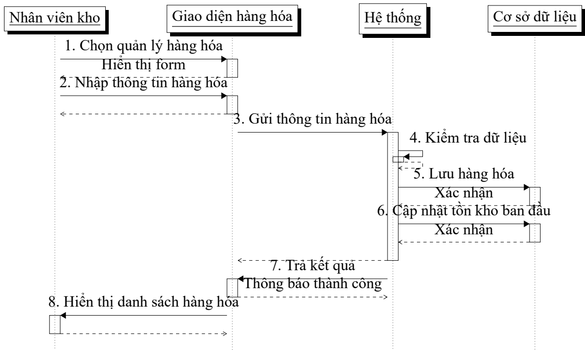
Hình 5.1: Sequence diagram UC05 – Quản lý hàng hóa
