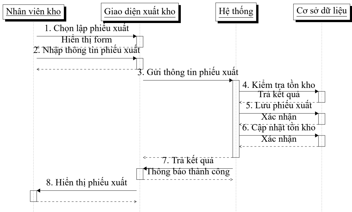
Hình 5.4: Sequence diagram UC10 – Lập phiếu xuất kho
