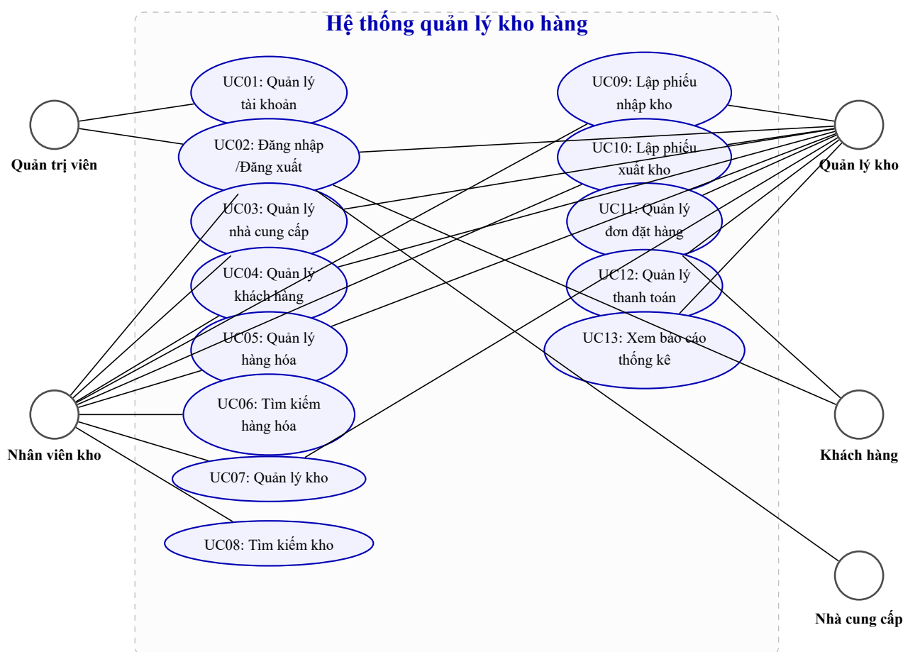
Hình 3.4: Sơ đồ use case tổng quát của hệ thống quản lý kho hàng
