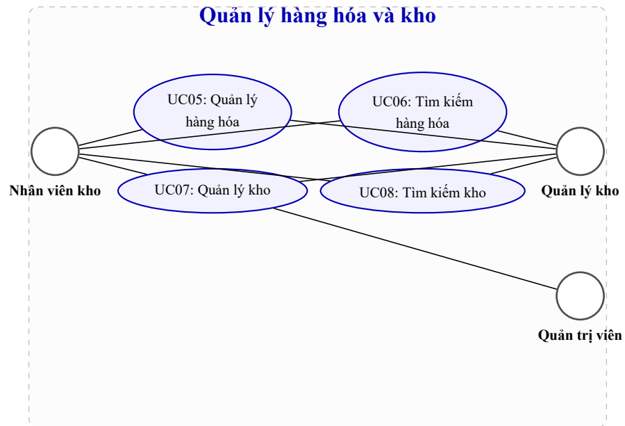
Hình 3.7: Sơ đồ use case phân rã – Quản lý hàng hóa và kho
