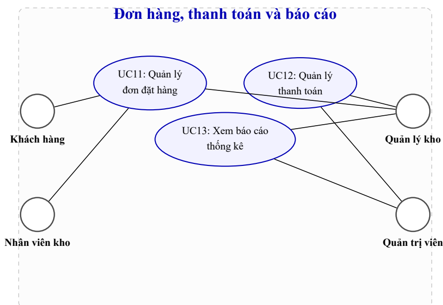
Hình 3.9: Sơ đồ use case phân rã – Đơn hàng, thanh toán và báo cáo
