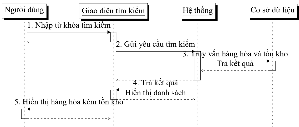
Hình 5.2: Sequence diagram UC06 – Tìm kiếm hàng hóa
